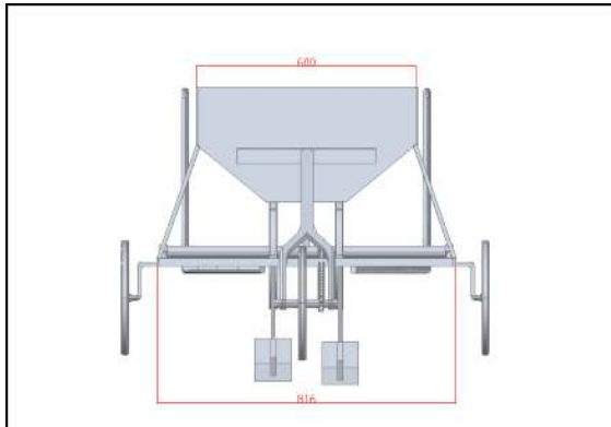
Gambar 3.8 Tampak Depan.
